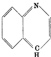
Chinolin.
